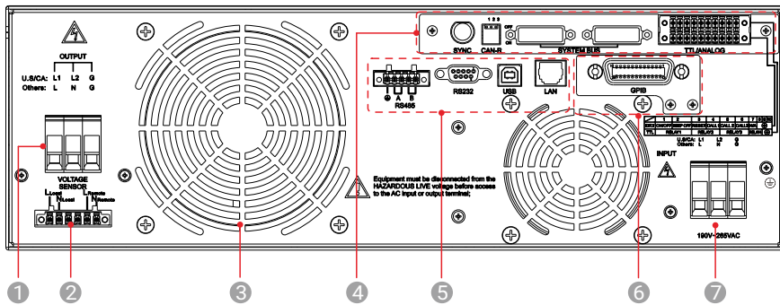
以3U机型后面板为例
