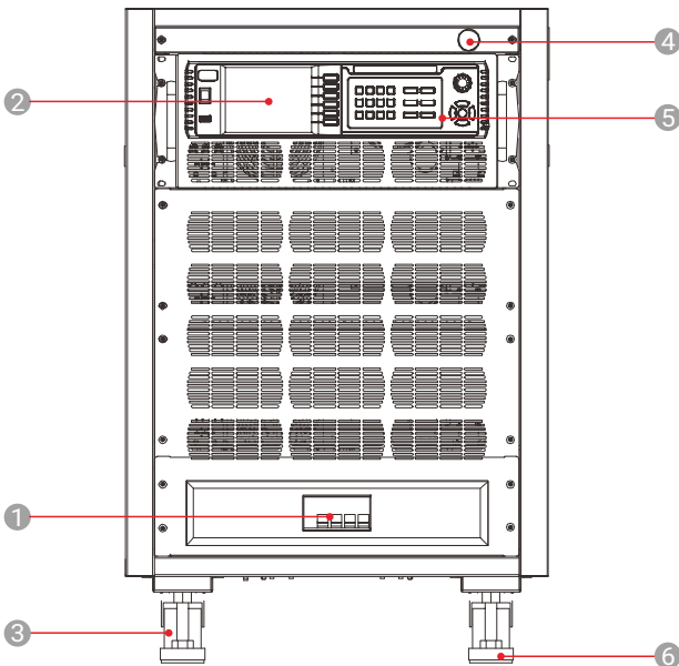
17U机柜前面板
