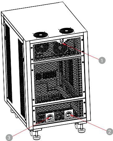
① 通讯线缆出线孔 ② 输入线缆入线孔 ③ 输出线缆出线孔
