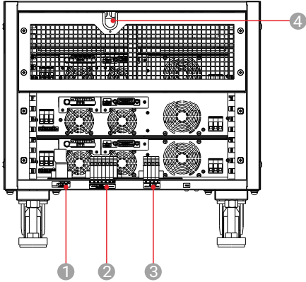
9U机柜后面板
